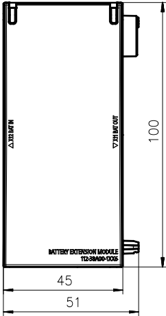
Vorne / Front
