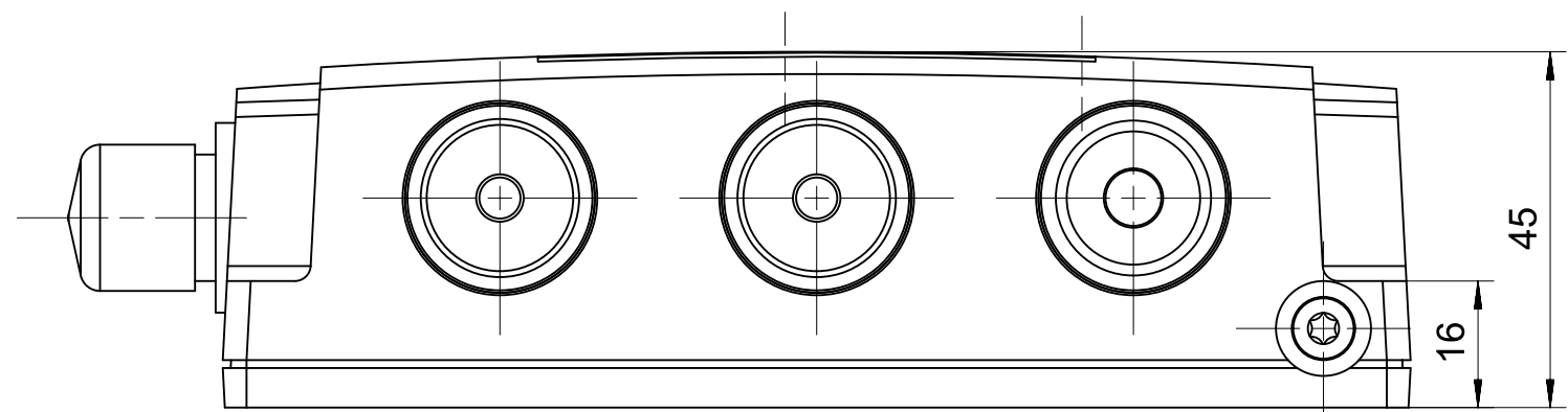
Unten / Bottom
