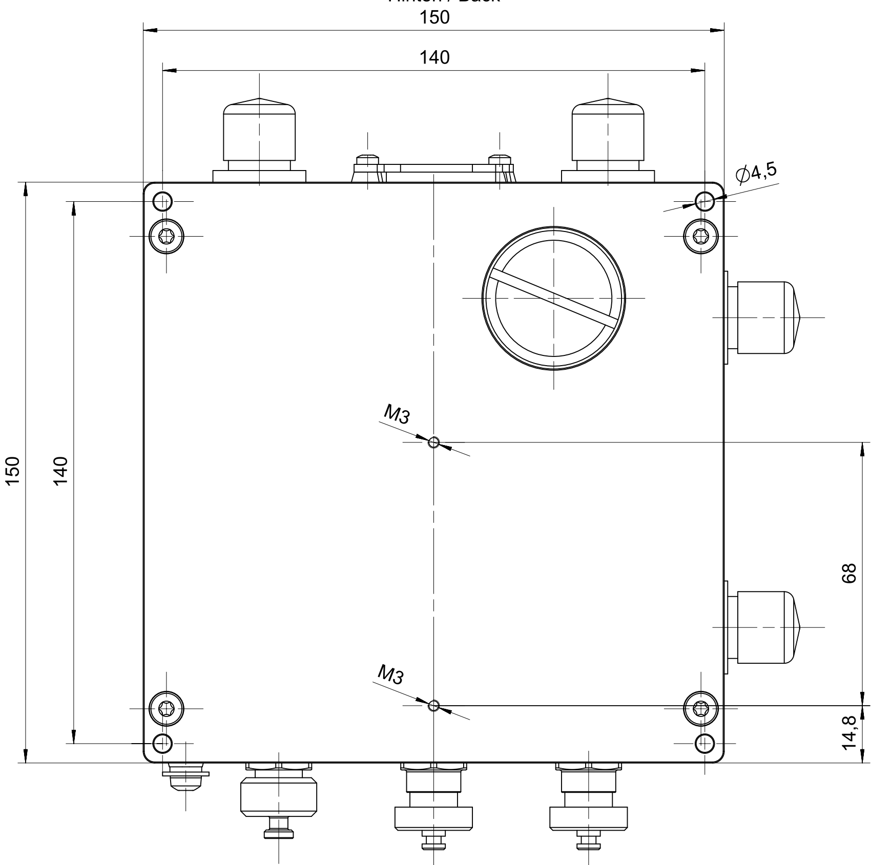
Hinten / Back
