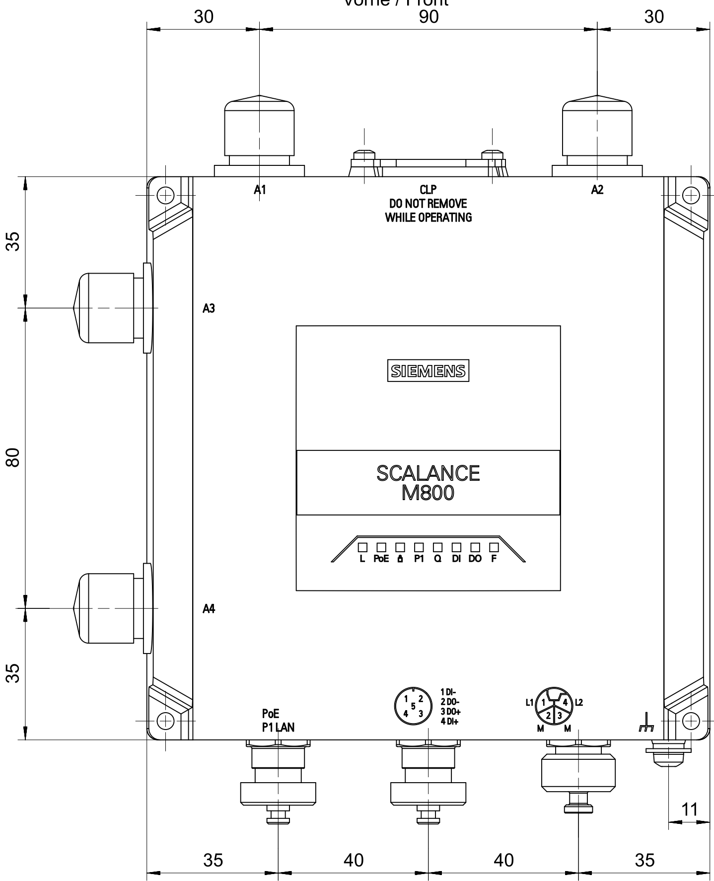
Vorne / Front
